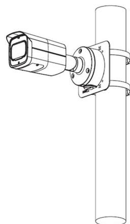
PFA135+PFA152-E 立柱安裝
